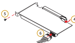
图2-9 显卡安装
