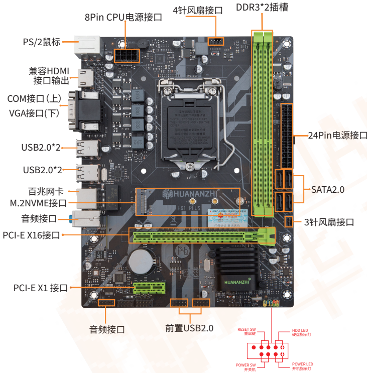
图1-1 H61 PLUS主板图解
